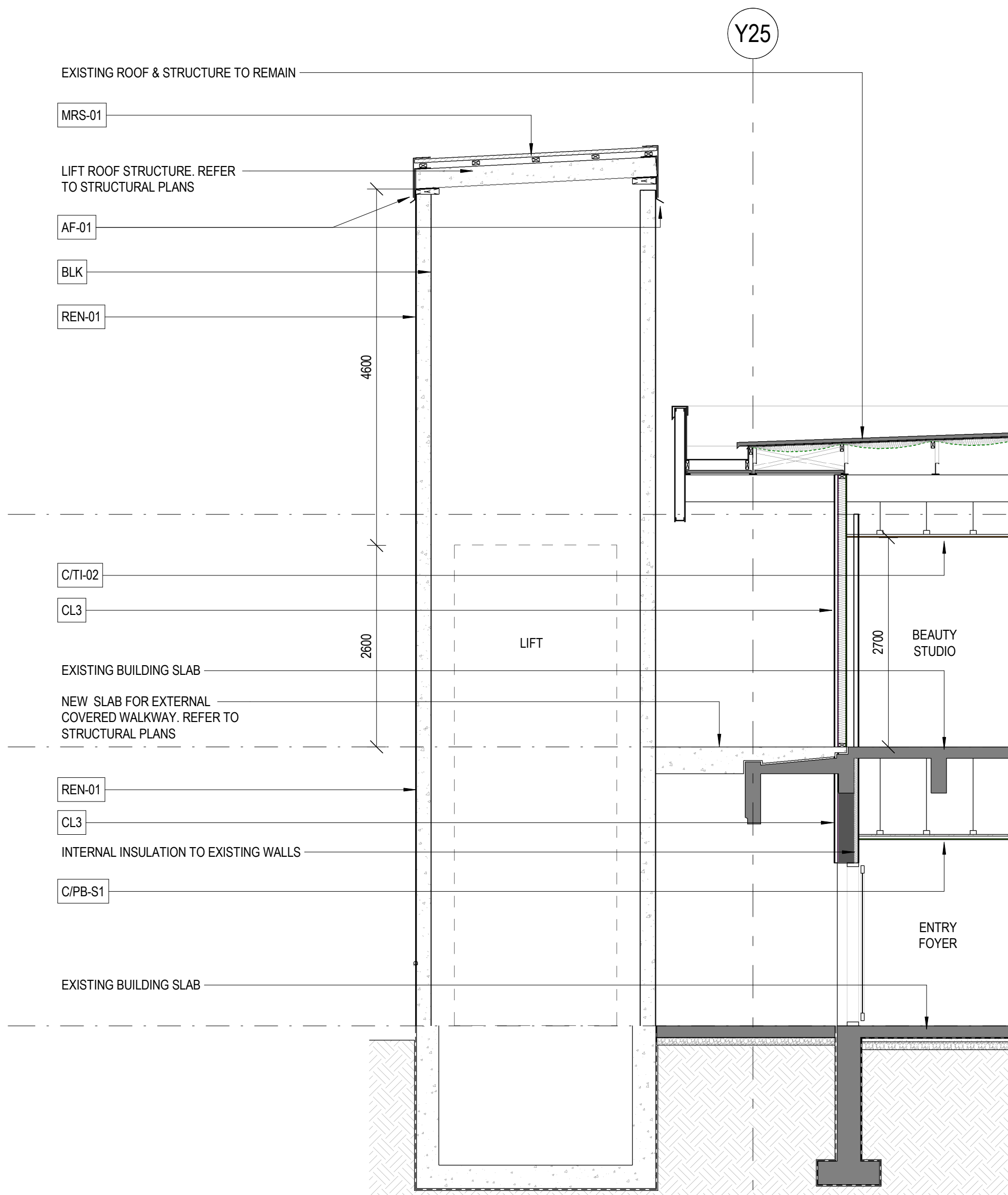
1 WALL SECTION 2 21-01 1 : 50
