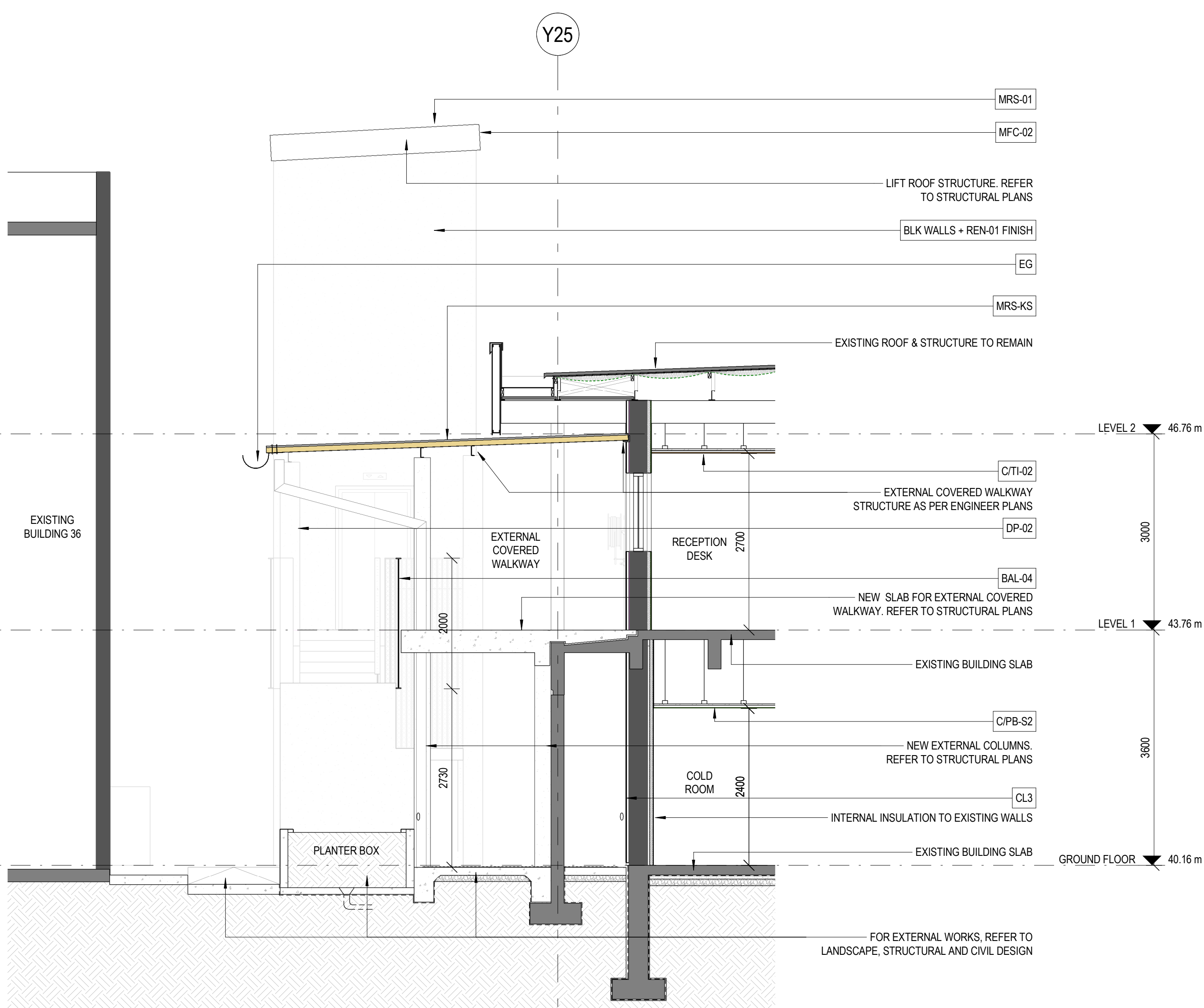
2 WALL SECTION 3 21-01 1 : 50
